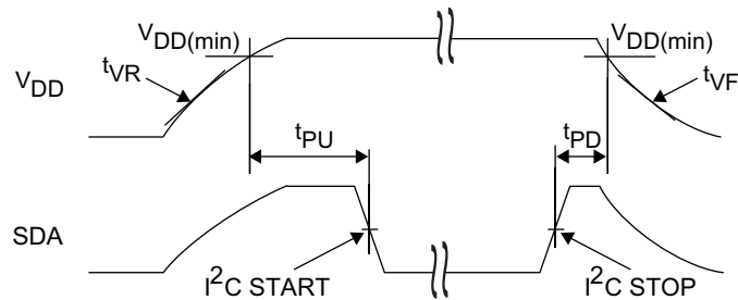
图 15. 电源时序
